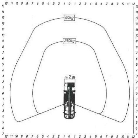
Stabilizzatori chiusi
