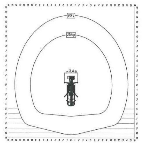
Stabilizzatori aperti
